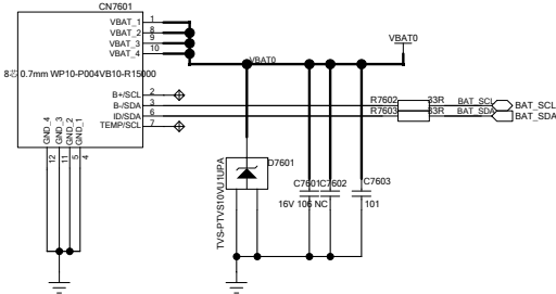
8Pin Battery Con
